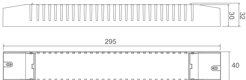
Dimension(mm)
